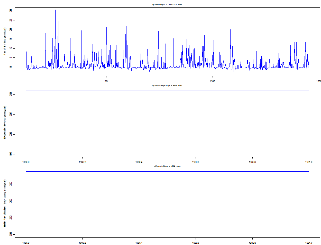
Figuur 28: PearlLysimeter
