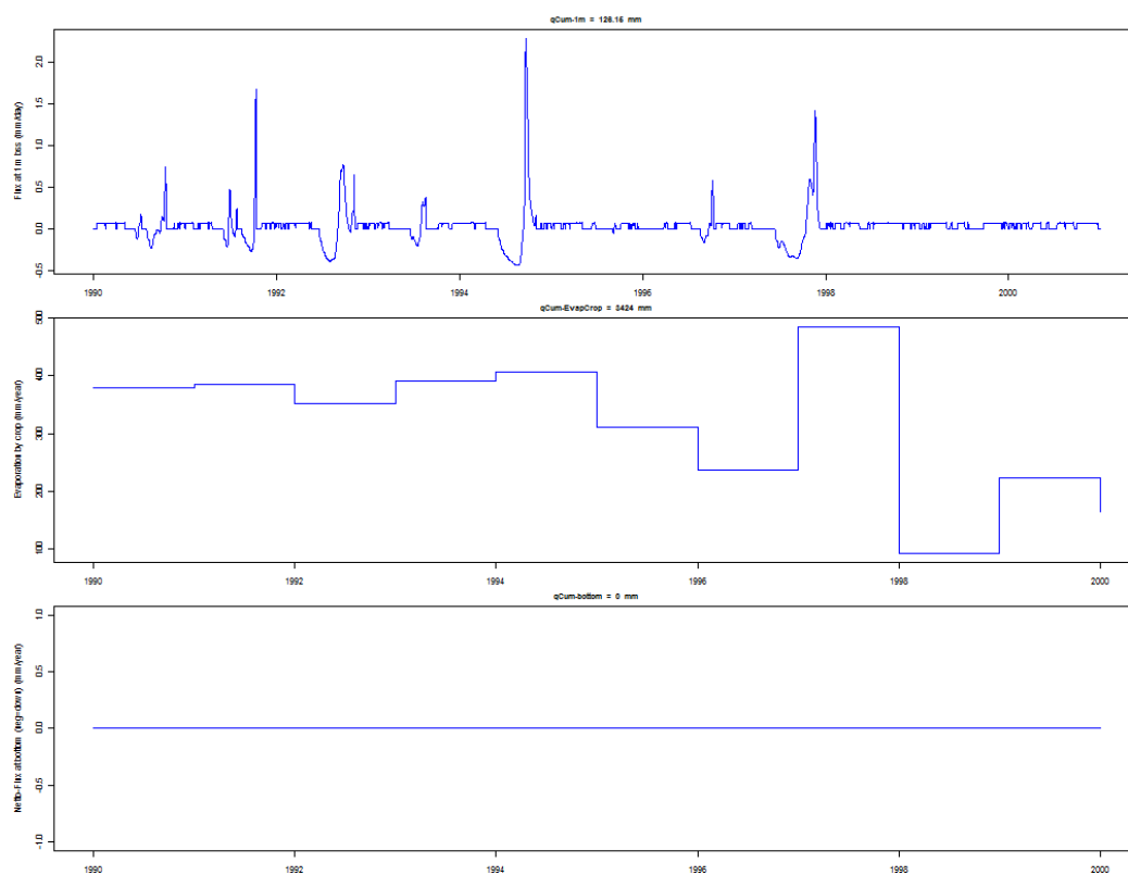
Figuur 31: SnowFrost(EuroHarpNOV)
