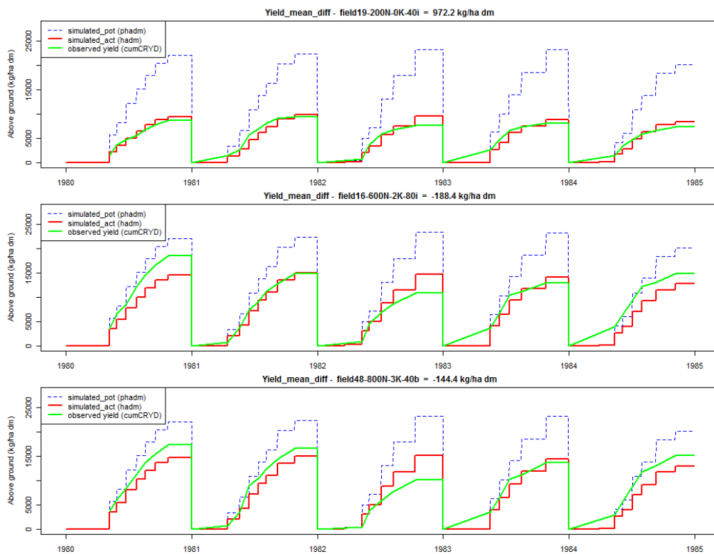
Figuur 35: CropgrowthGrassland(Ruurlo)
