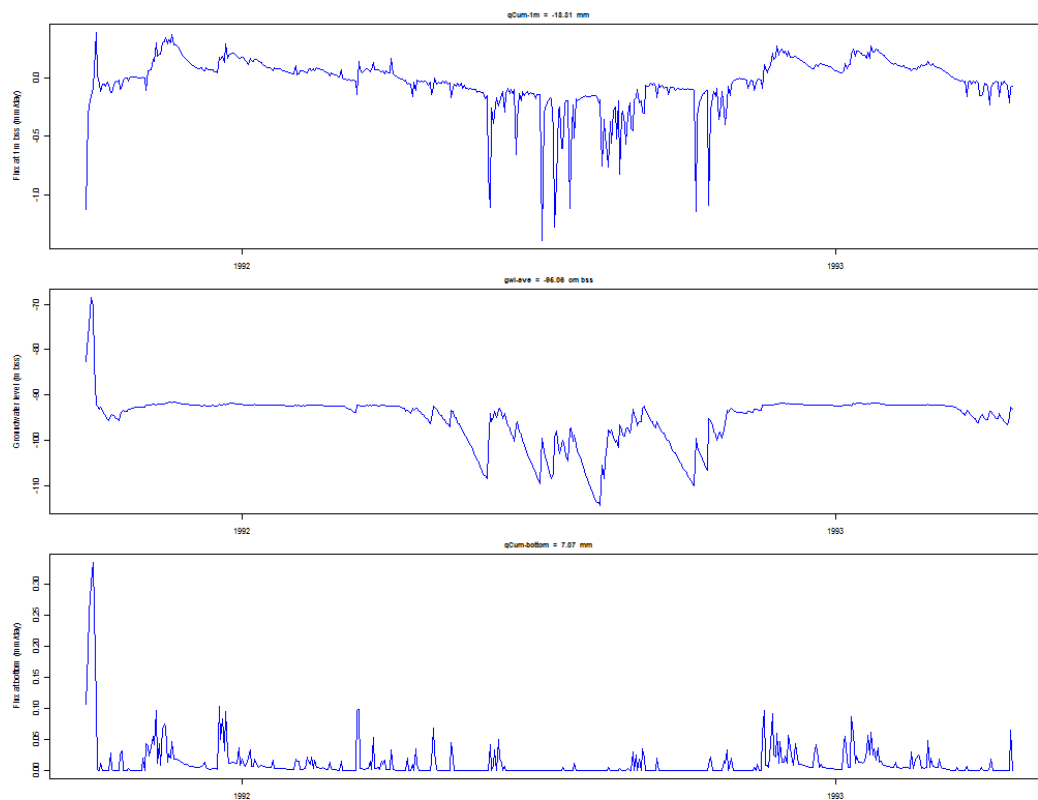
Figuur 20: MacroPores2
