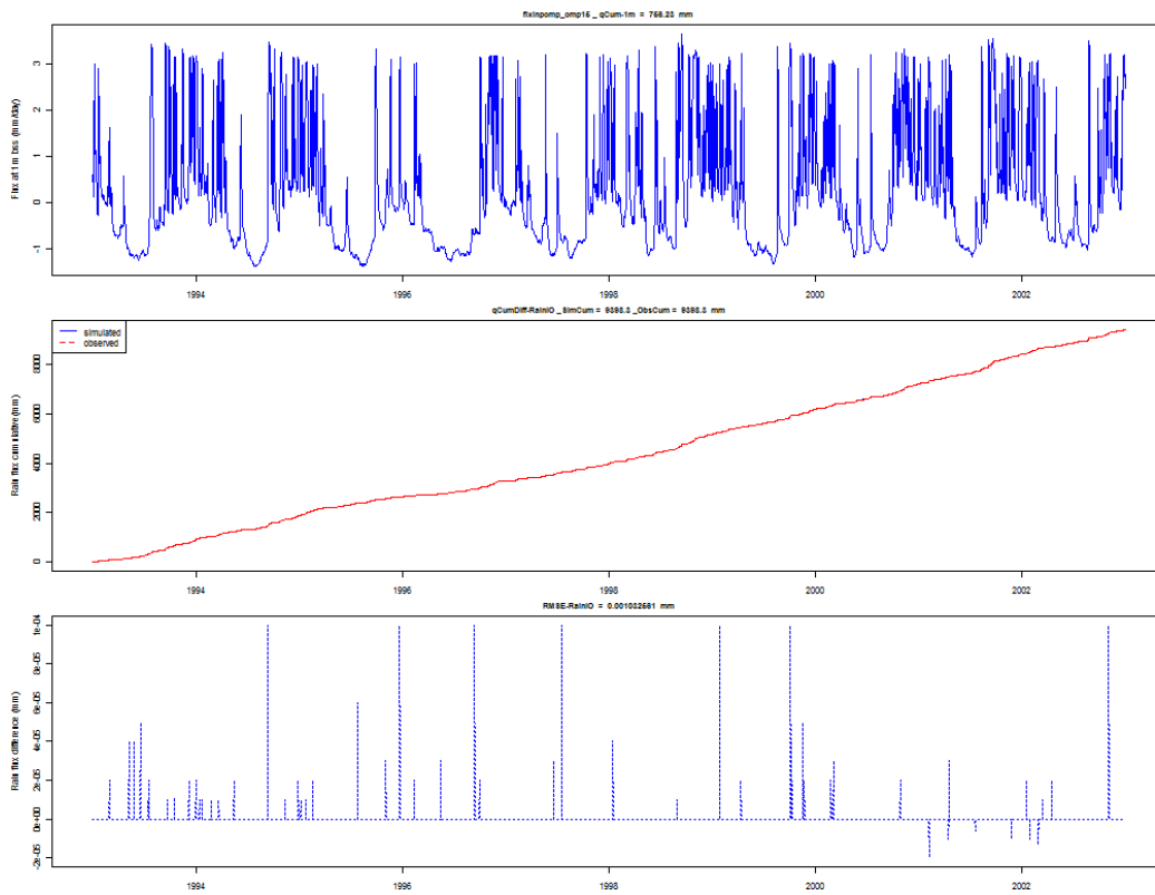
Figuur 13: GwlShallow(Zegveld)
